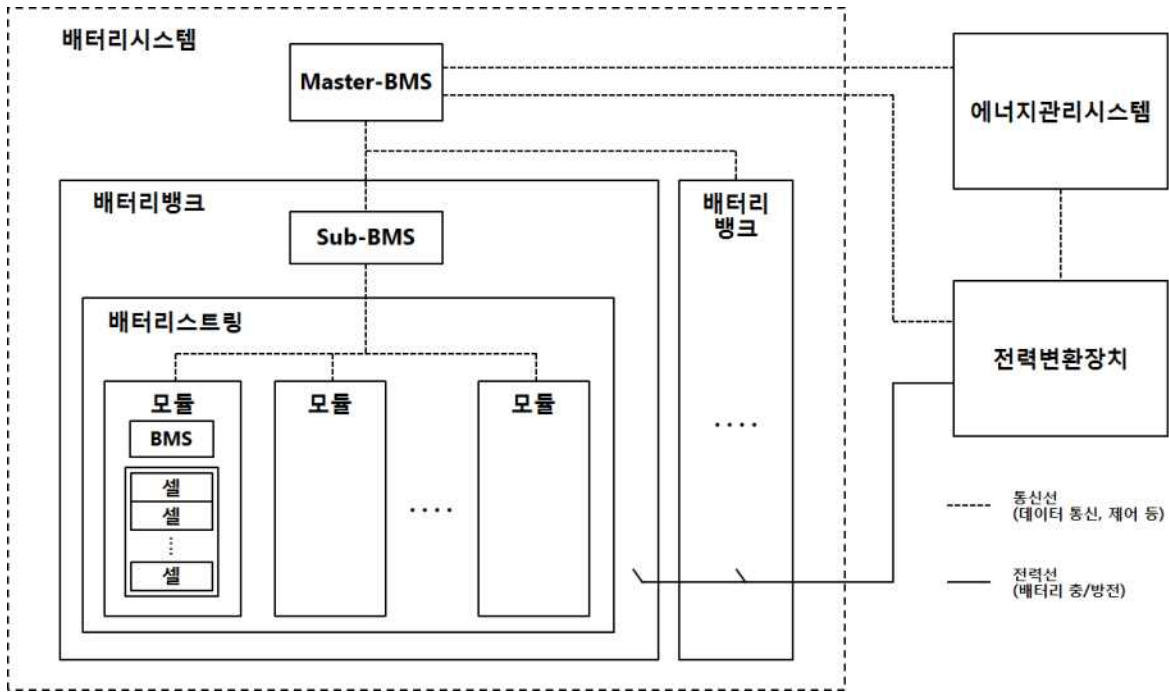
그림 1 배터리시스템 구성도 (2019)
