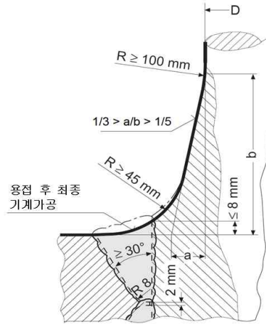
그림 4.1.6 타두재와 커플링 플랜지 간의 용접고착
