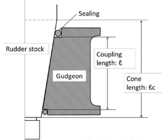
그림 4.1.7b 콘 길이 및 커플링 길이
