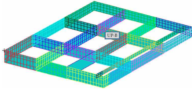
그림 4.2.8 창구덮개 1차 지지부재의 웹
