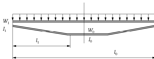
그림 4.2.5 단면이 변하는 1차 지지부재
