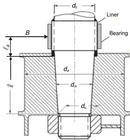
그림 4.1.9 핀틀 콘커플링 \ell_a
