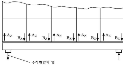
그림 4.2.13 창구덮개의 수직방향 힘
