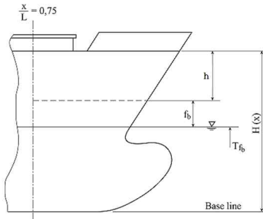
그림 4.2.11 H(x) 의 정의
