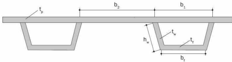
그림 4.2.6 U형 보강재가 시공된 창구덮개의 예
