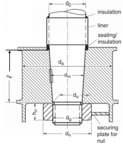
그림 4.1.7 키를 가지는 콘커플링
