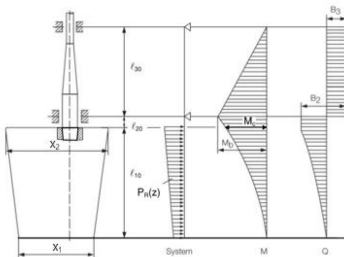
그림 4.1.2 C형 타(스페이드 타)
