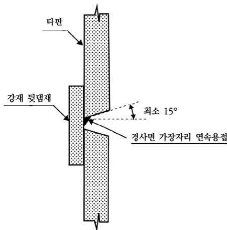
그림 4.1.2 타판의 강재 뒷담재를 사용한 완전용입용접
