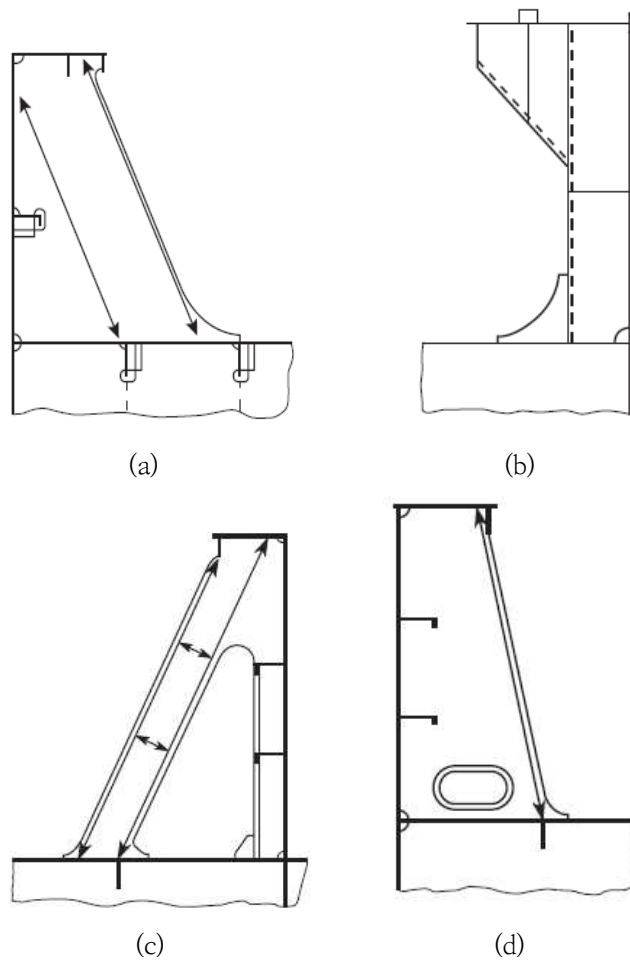
그림 4.2.9 일반적인 창구코밍 스테이
