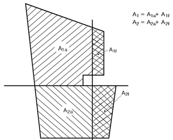
그림 4.1.4 타면적의 분할
