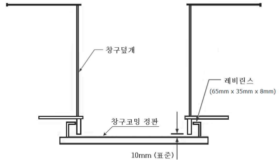
그림 4.2.12 레비린스의 예
