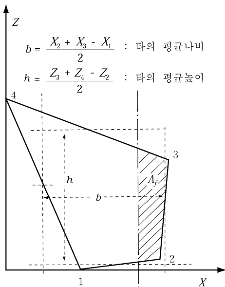
그림 4.1.3 타의 좌표계
