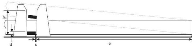
그림 4.2.14 창구덮개 횡방향 가이드 높이
