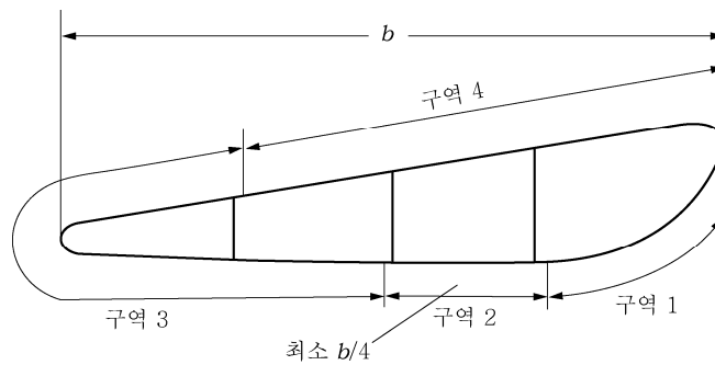
그림 4.1.10 프로펠러 구역
