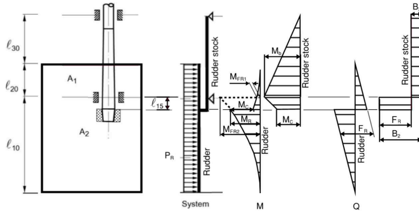
그림 4.1.3(가)
