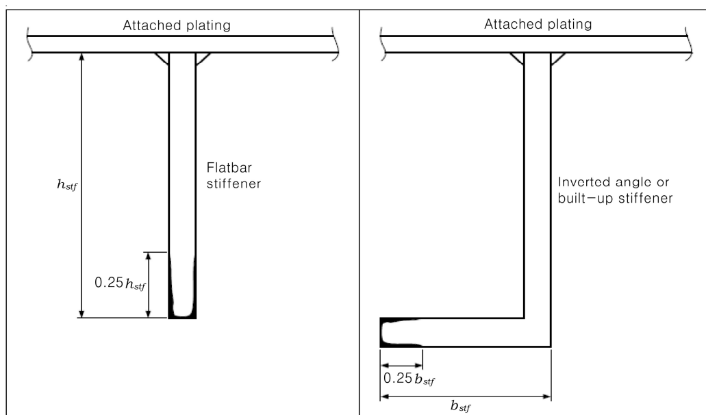
Fig 1.2.4 Edge corrosion
