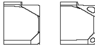
그림 3-1 Bulk Carrier 'ESP'의 중앙횡단면 예
