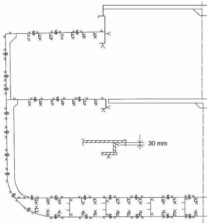
그림 5 일반선박의 계측위치
