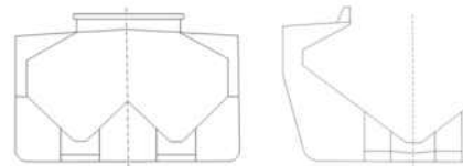
그림 3-2 Self-Unloading Bulk Carrier 'ESP'의 중앙횡단면 예
