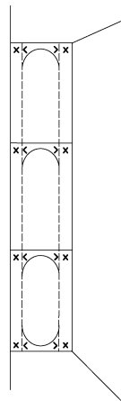
그림 8 이중선체 산적화물선의 이중선체측탱크 횡늑골에 대한 계측위치
