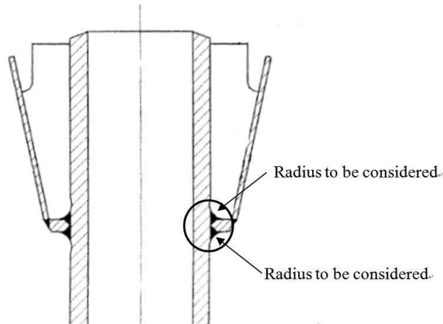
그림 3.2.7 용접 곡률반경
