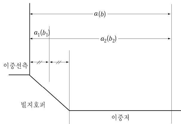
그림 3.3.6 a_1, a_2, b_1 및 b_2 의 측정
