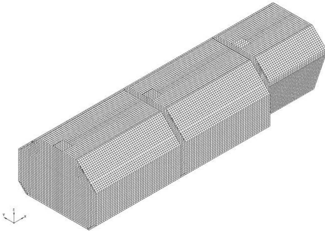
그림 33 화물창 모델의 예(Mark III 형식, 선체외곽부재 제외)
