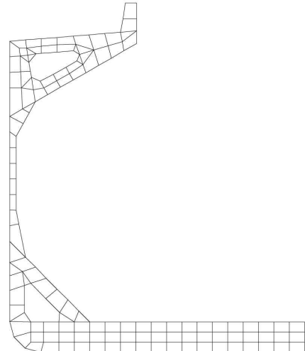
그림 11 Web frame 모델의 예
