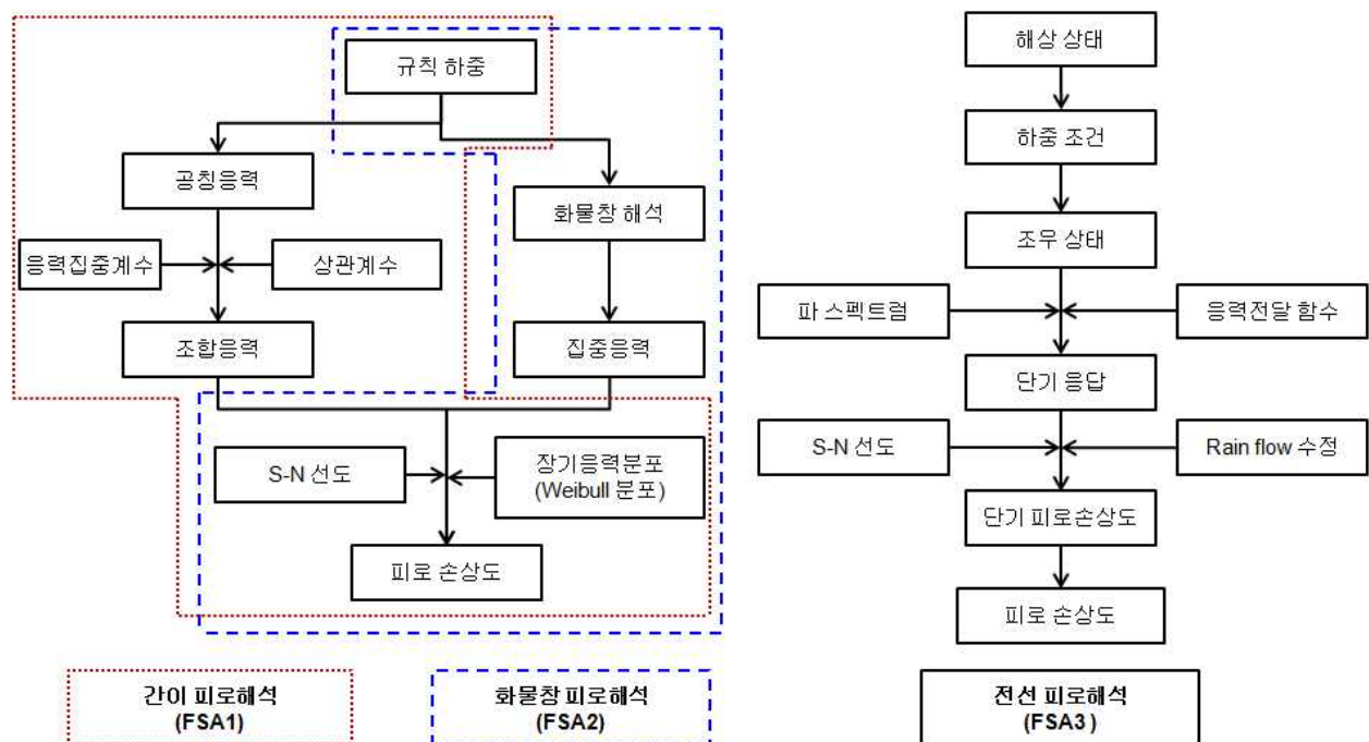
그림 1 피로해석 방법
