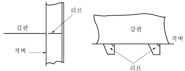
그림 3.14.4 리브
