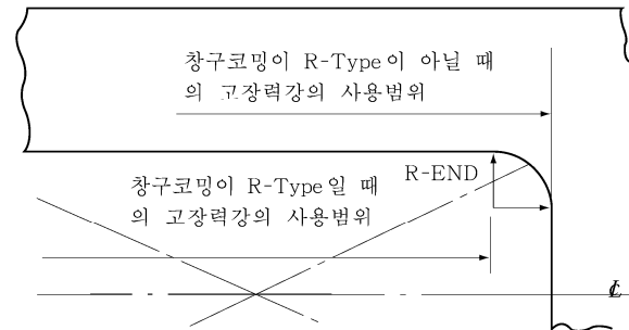
그림 3.1.8 창구코밍
