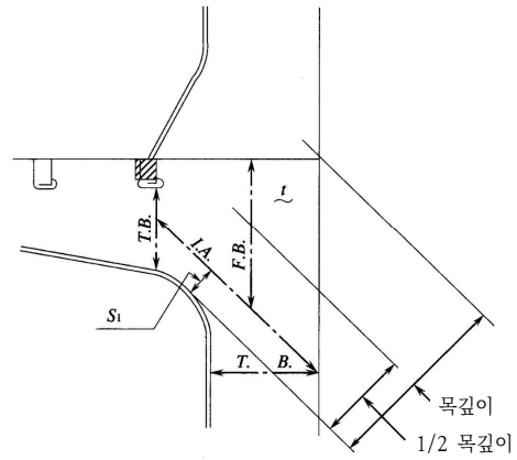
그림 3.9.4 브래킷의 보강
