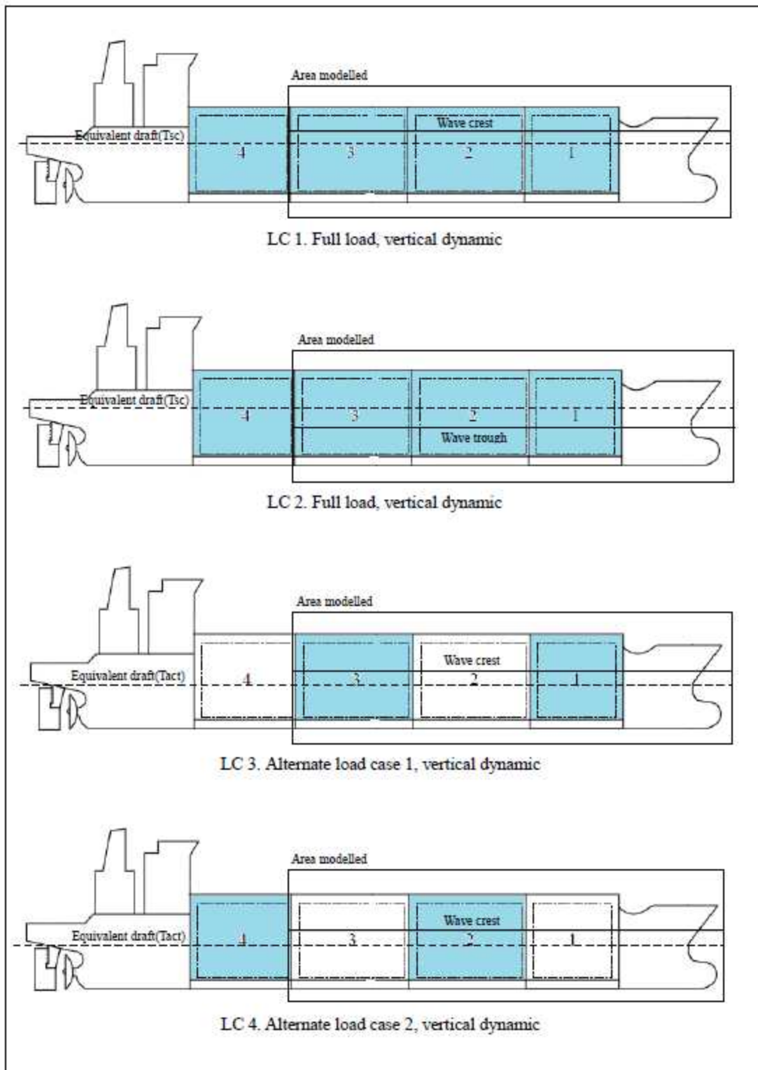
그림 46 하중 조건(표 40 참조) (2018)
