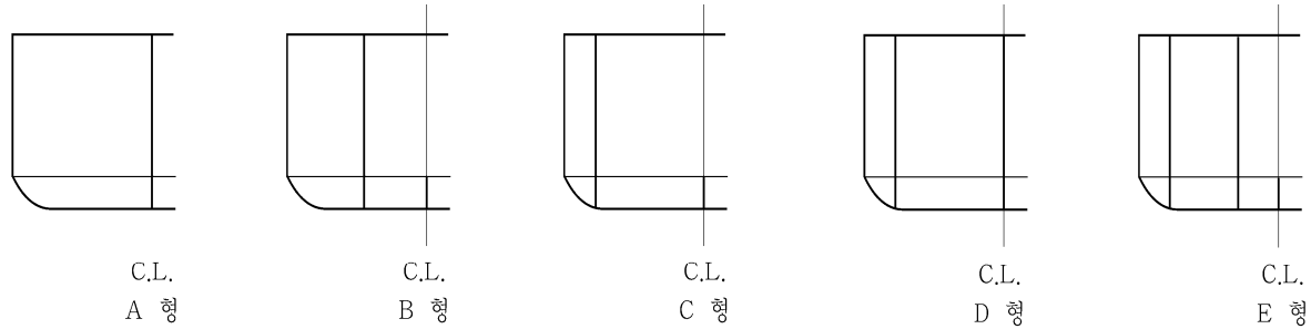
그림 3.3.7 종격벽 배치에 따른 선박의 분류
