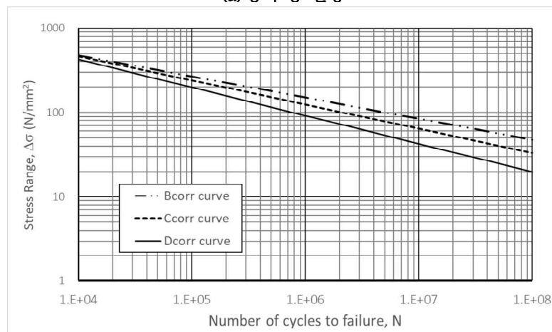
그림 2 설계 S-N 선도 (2020)
