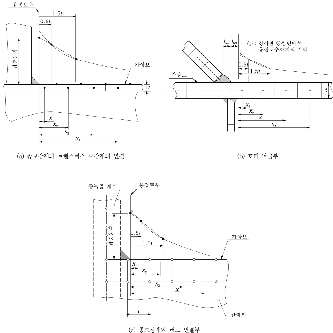
그림 5 집중응력 산정방법
