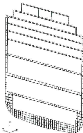
그림 28 특설늑골의 예
