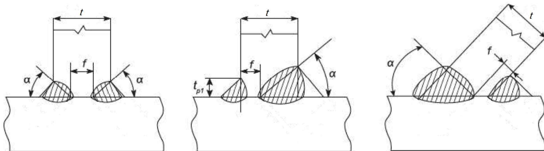
그림 3.1.2 부분용입용접
