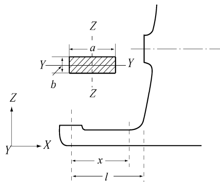
그림 3.2.1 슈피스의 좌표
