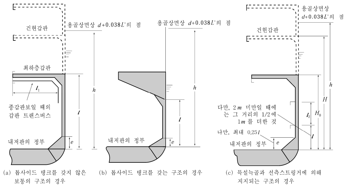
그림 3.8.2 선창내 늑골에 대한 l , h 및 H 등의 측정방법
