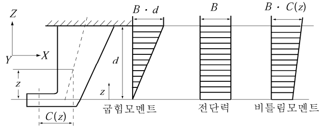
그림 3.2.2 리더혼의 하중
