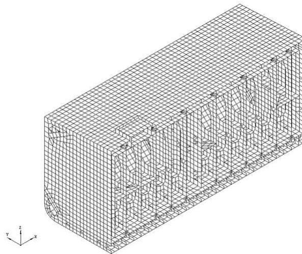
그림 51 화물창 모델 예(중양부 화물창, 중심선 단면 표시)
