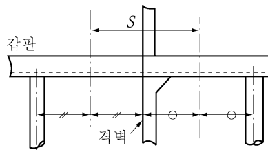
그림 3.14.2 S의 측정방법
