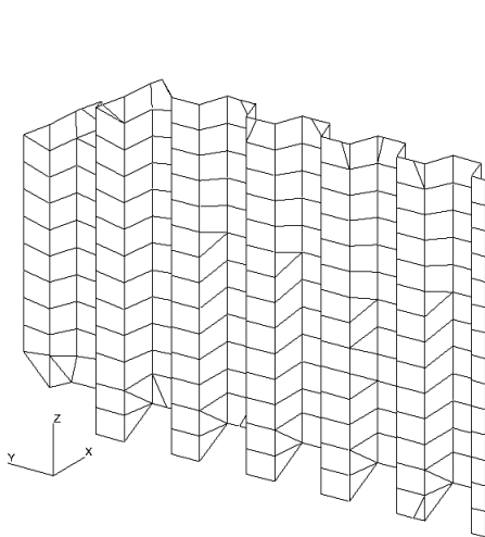
그림 10 파형격벽 모델의 예
