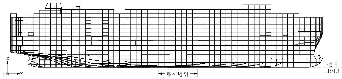
그림 26 해석범위
