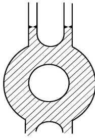
그림 3.2.3 프로펠러 보스와 강의결합
