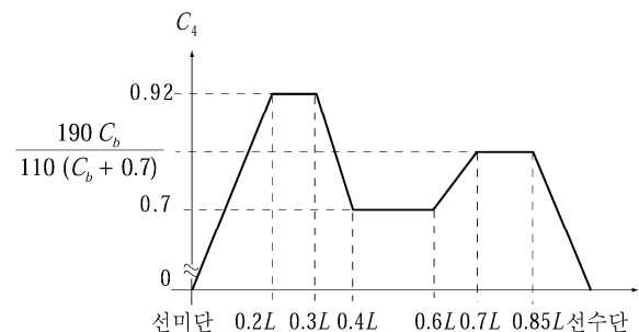
그림 3.3.6 계수 C_4 의 값
