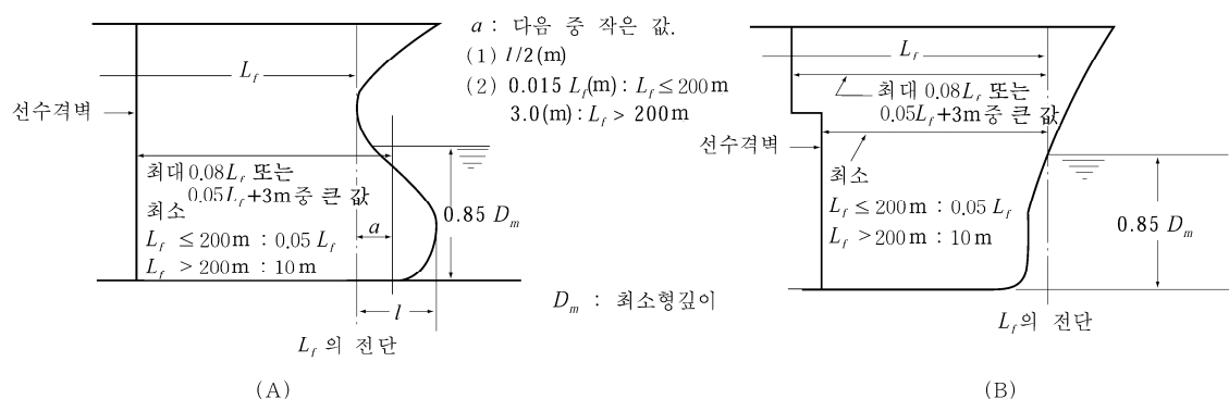
그림 3.14.1 선수격벽의 위치측정방법
