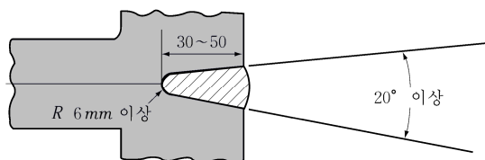
그림 3.2.1 주강선미재의 상호 용접 이음
