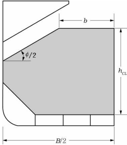
그림 14 화물창의 적재형상
