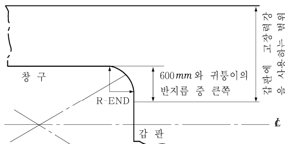
그림 3.1.7 갑판
