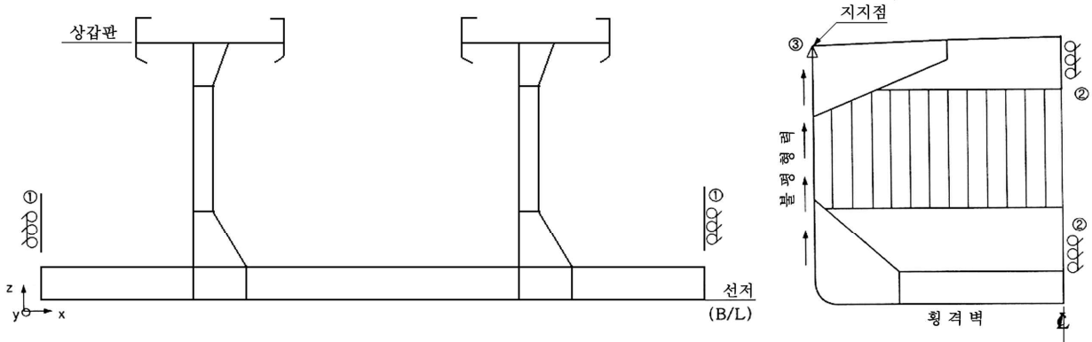
그림 13 경계조건
