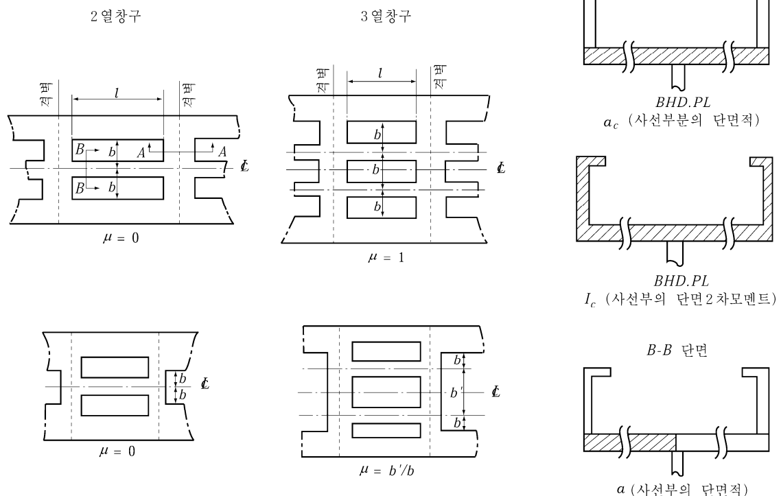
그림 3.3.2 l , b 및 \mu
