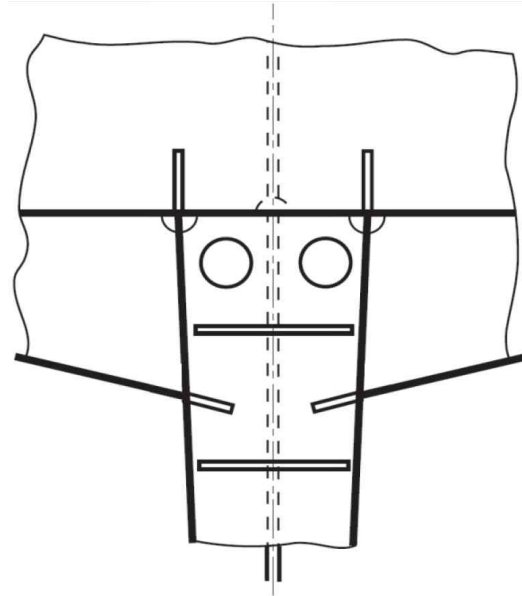
그림 3.2.6 러더혼과 선미구조의 결합
