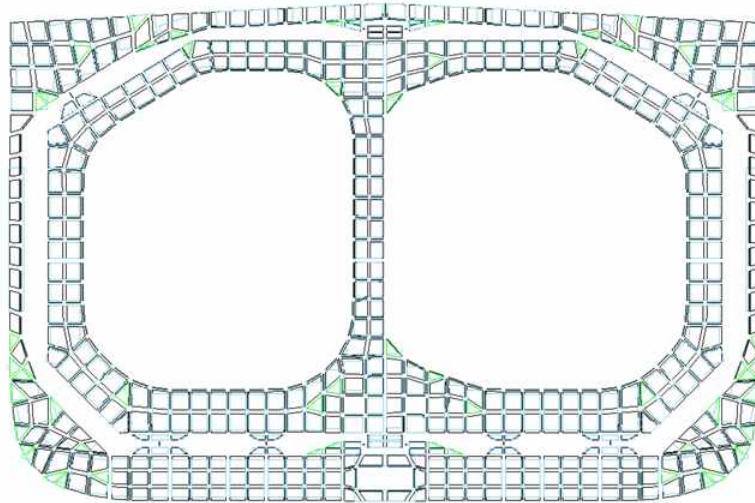
그림 48 횡단면
