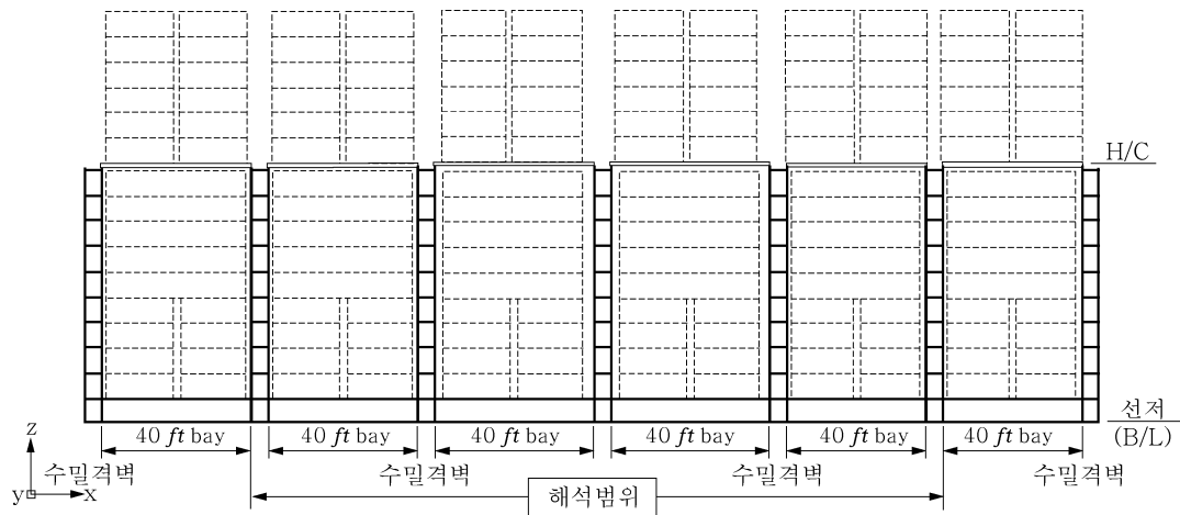
그림 19 해석범위
