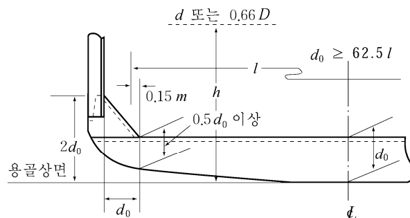
그림 3.6.1 늑판의 모양
