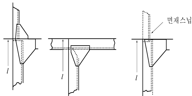
(a) 그림 3.14.2 끝부분의 고착
