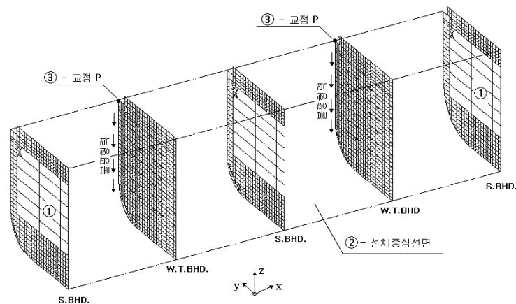
그림 24 경계조건 (대칭하중)
