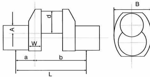
그림 5.6.15 공기압축기의 크랭크 스로우
