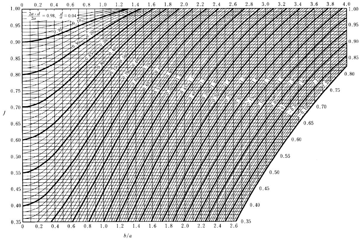
그림 5.5.3 관구멍이 경사진 방향으로 배치된 관구멍부의 리가먼트 효율
