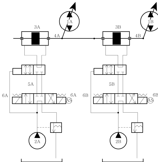
(b) 기계적으로 결합된 장치
