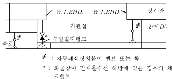
그림 5.6.8 수밀격벽에 단이 있는 경우의 선창의 발지배수의 예
