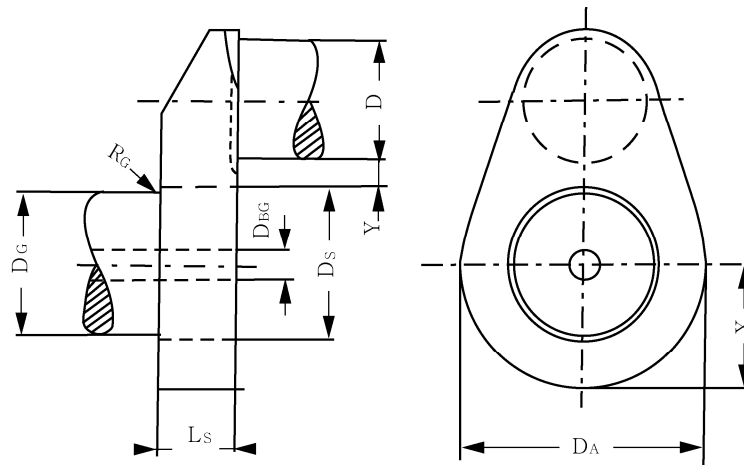
그림 6 반조립형 크랭크축의 크랭크 스톱
