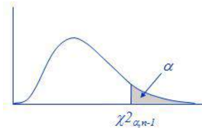
그림 13 카이제곱분포(chi-square distribution)
