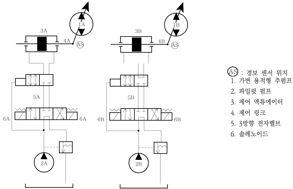
(a) 분리된 장치
