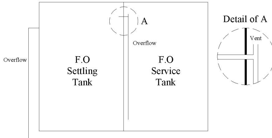
그림 5.6.4 넘침관의 상세
