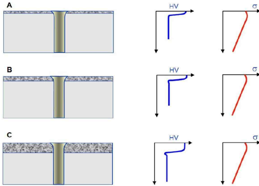
그림 20 고주파경화 오일구멍에서의 응력 및 정도
