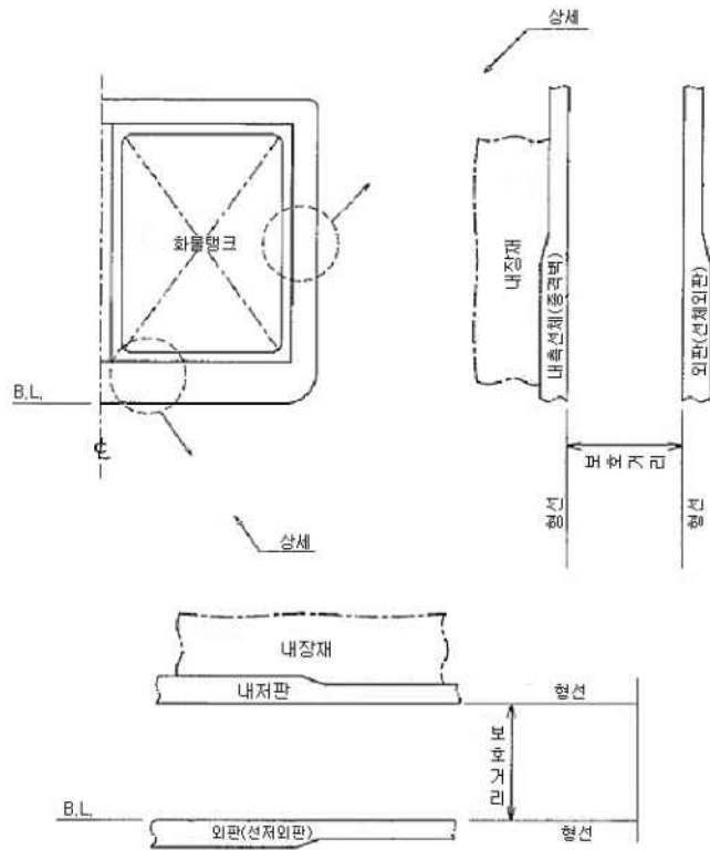
그림 7.5.1 (a) - 보호거리 (독립형 주형탱크)
