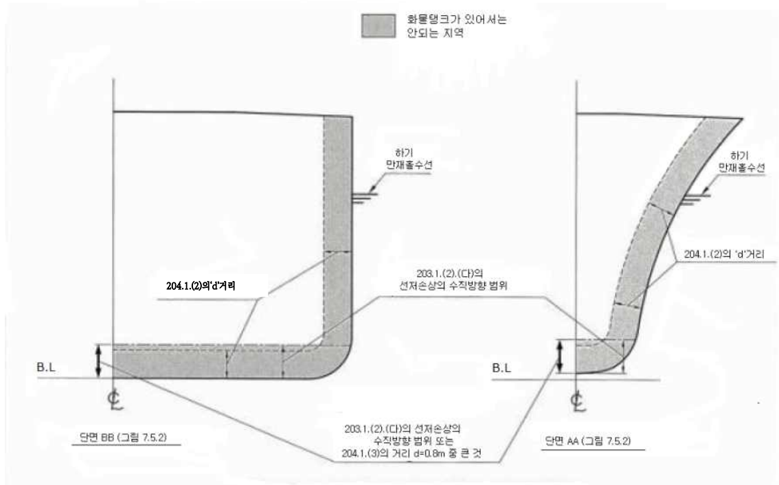
그림 7.5.4 탱크위치의 요건 (횡단면-2G 및 2PG형 선박)
