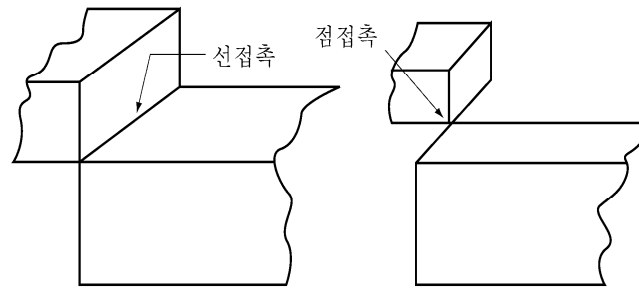
그림 7.5.8 2차 방법을 가진 화물창 구역의 격리
