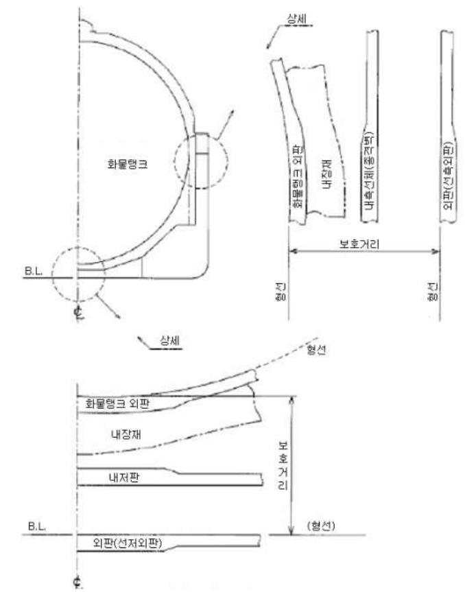
그림 7.5.1 (d) - 보호거리 (구형 탱크)
